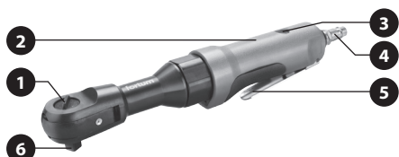
Abb. 2, Ratschen-Schlagschrauber Fortum®4795015
